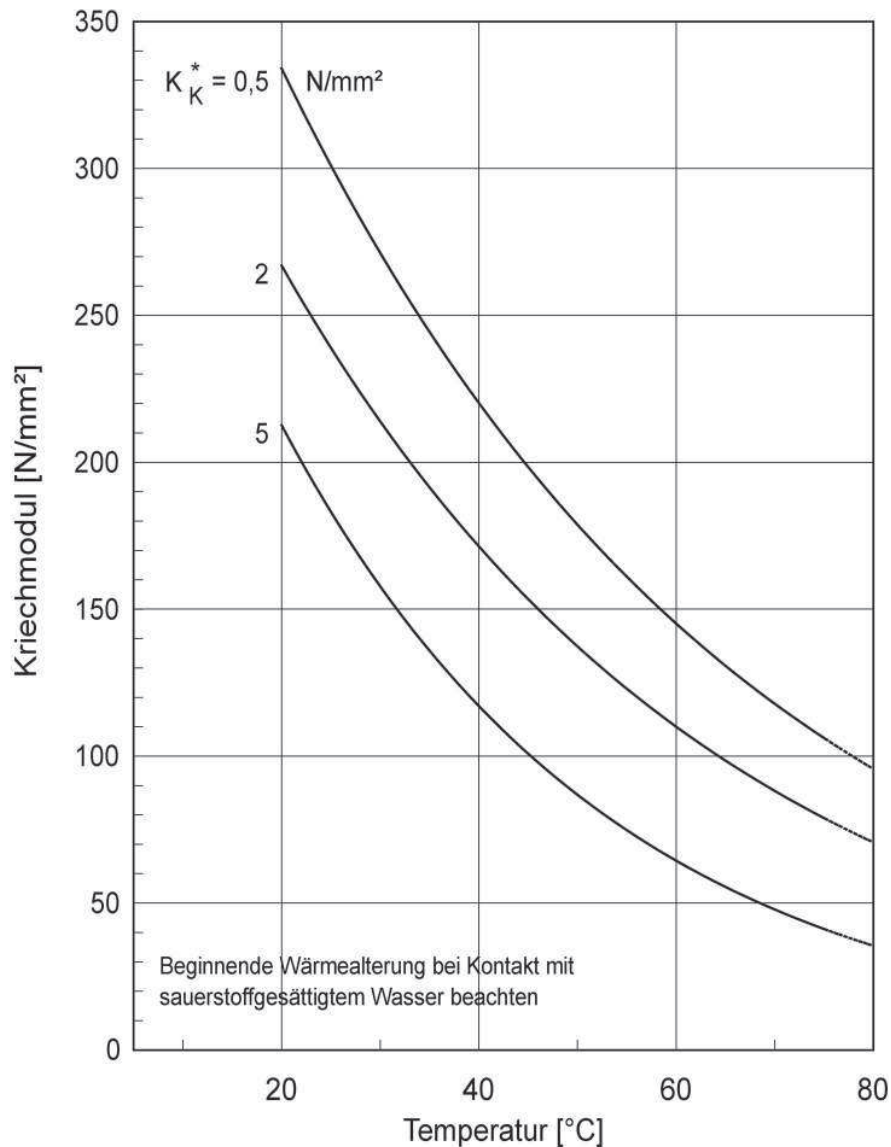
Bild 1. Kriechkurven von Polyethylen PE 80 für 1 Jahr.
